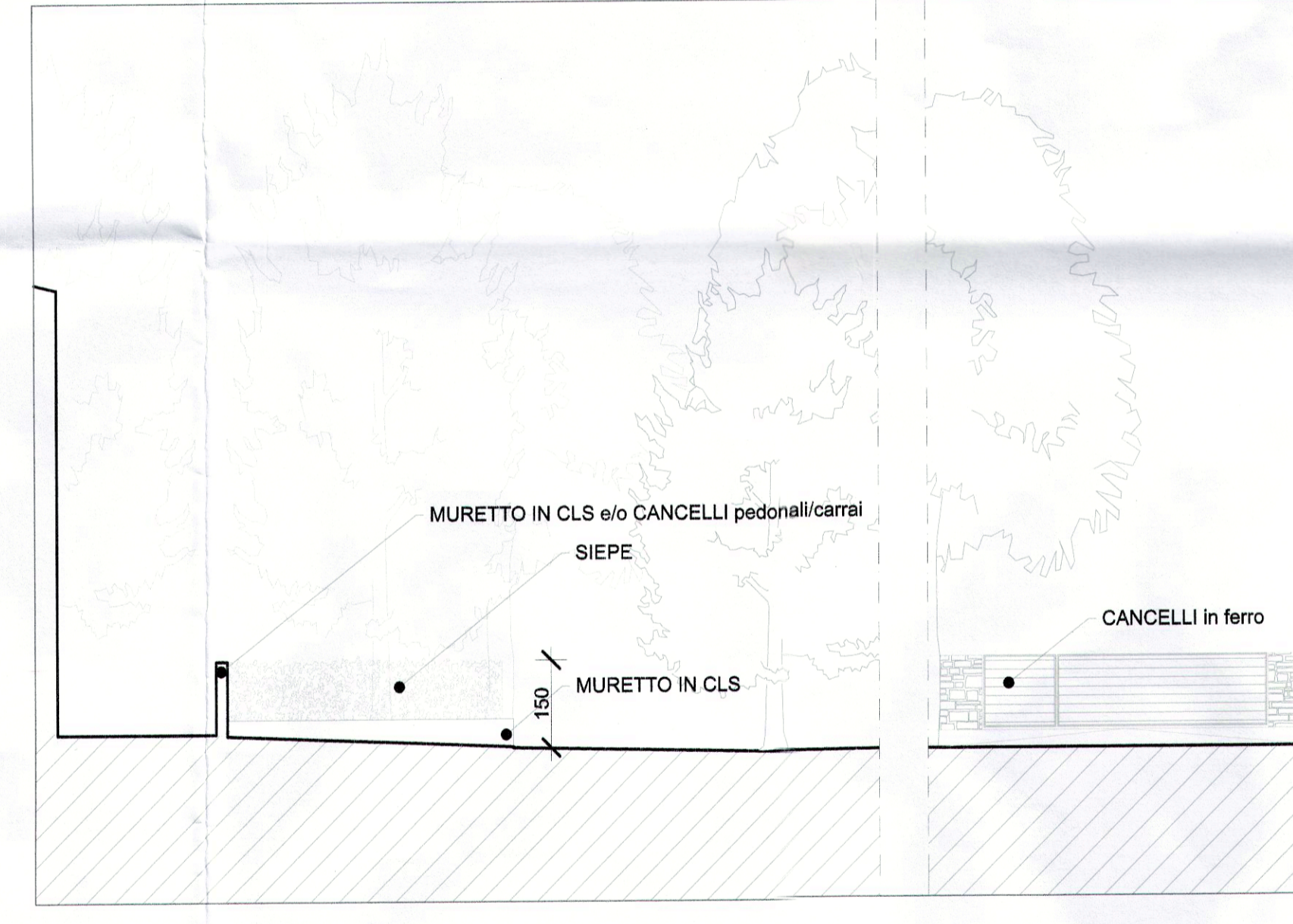
sezione D - D' (RECINZIONE tipo C) - scala 1:100
