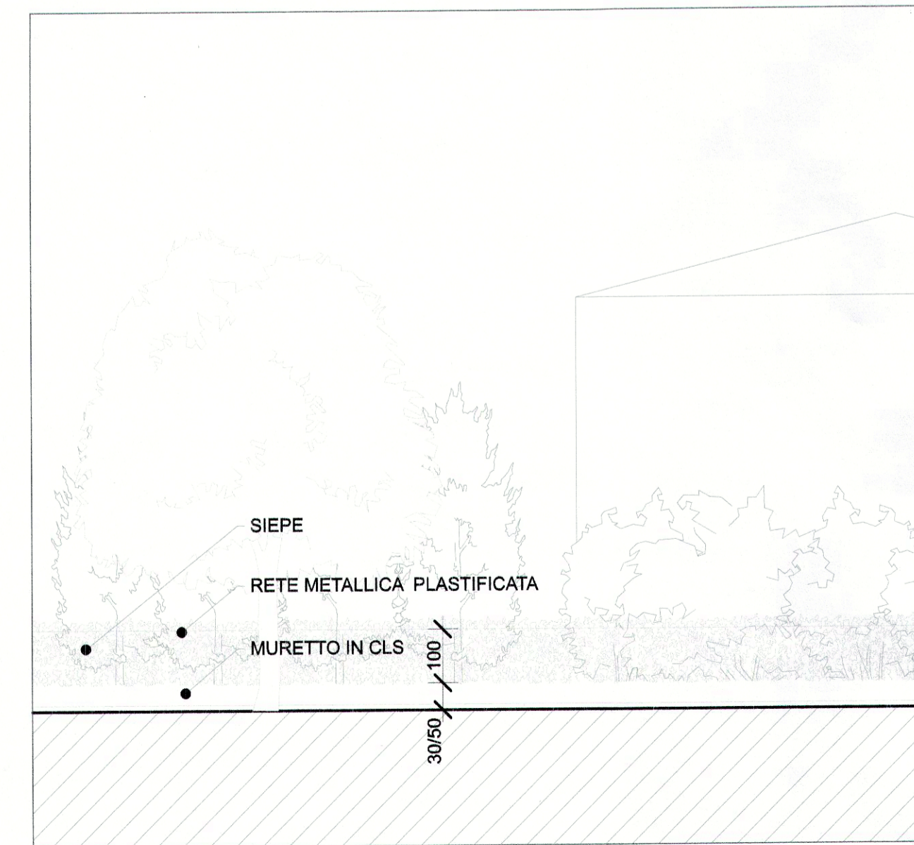
sezione E - E' (profilo INGRESSO) - scala 1:100
