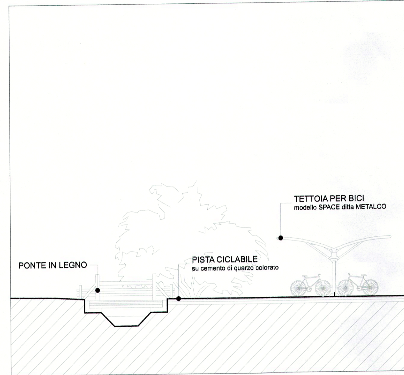
sezione X - X' - scala 1:100
