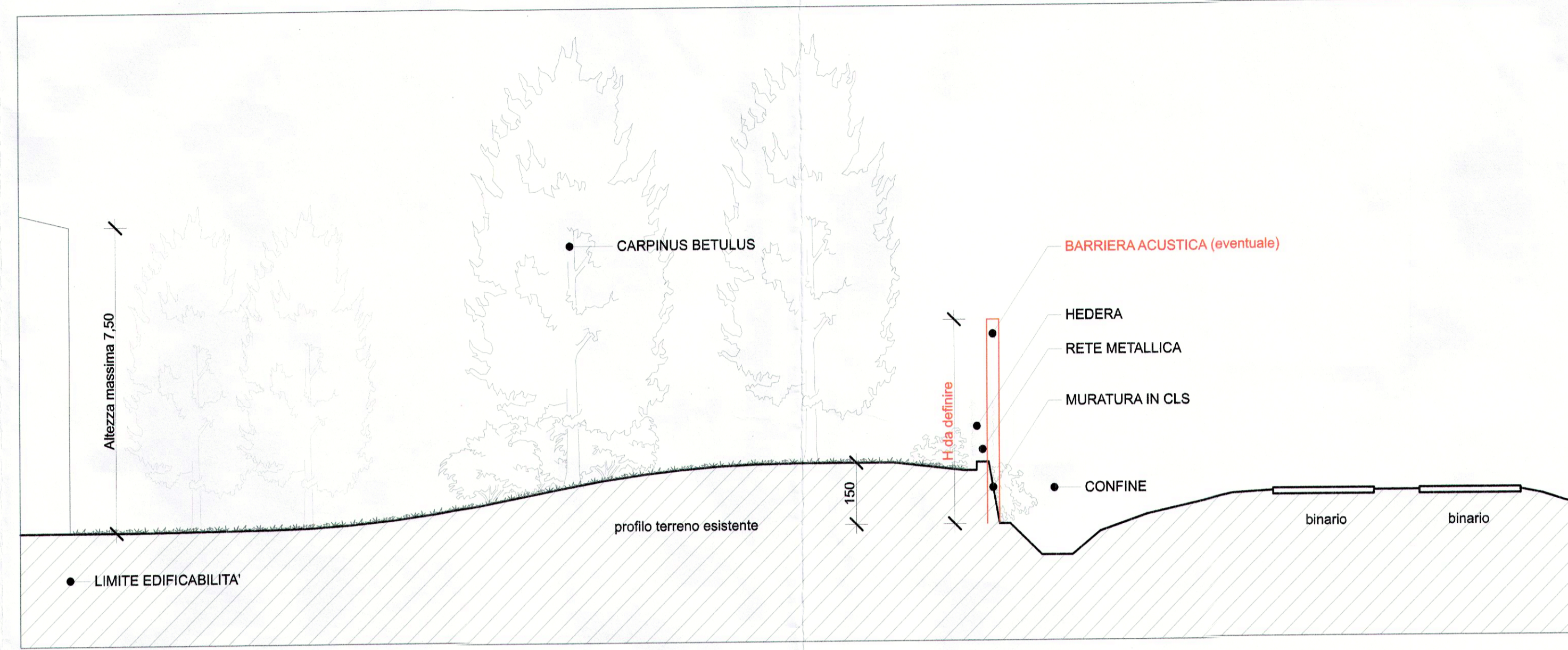
sezione Z - Z' - scala 1:100
