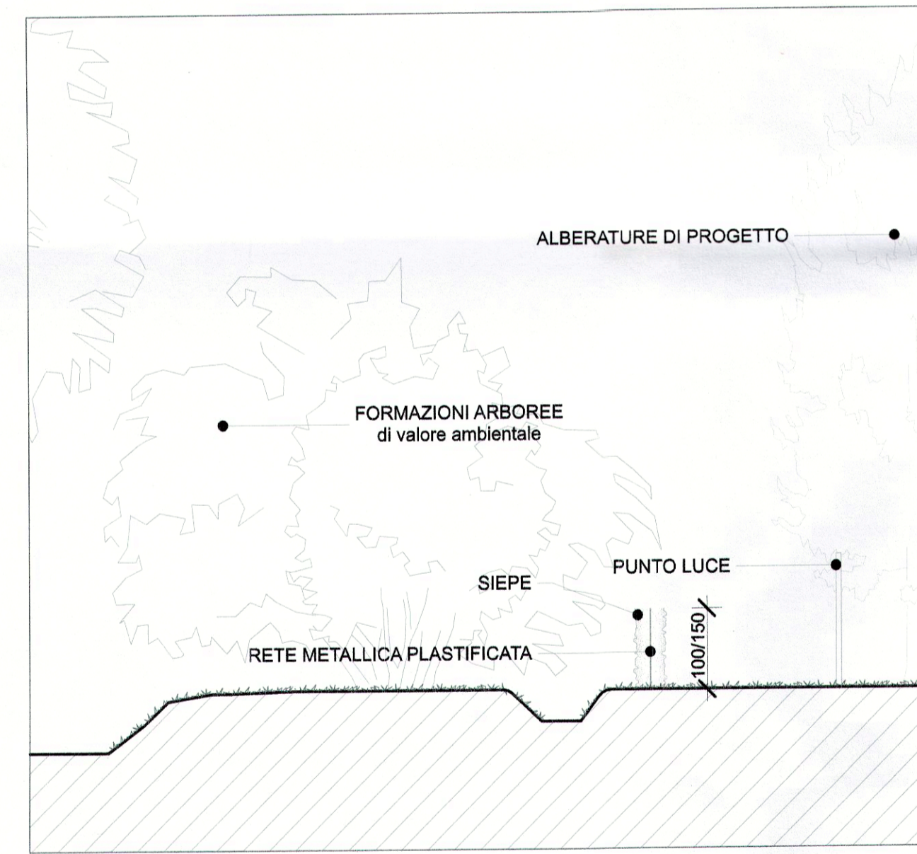
sezione B - B' (RECINZIONE tipo A) - scala 1:100
